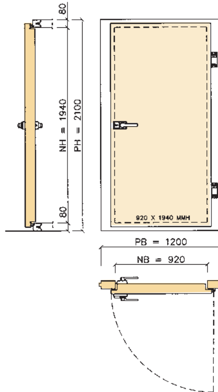
MDE 092/194 VÄNINGSDÖRR
