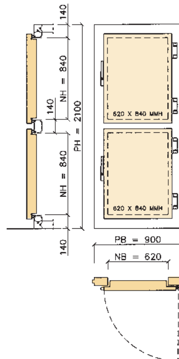
MDE 092/194 VÄNINGSDÖRR
