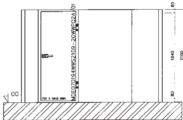
VOORAANZICHT
